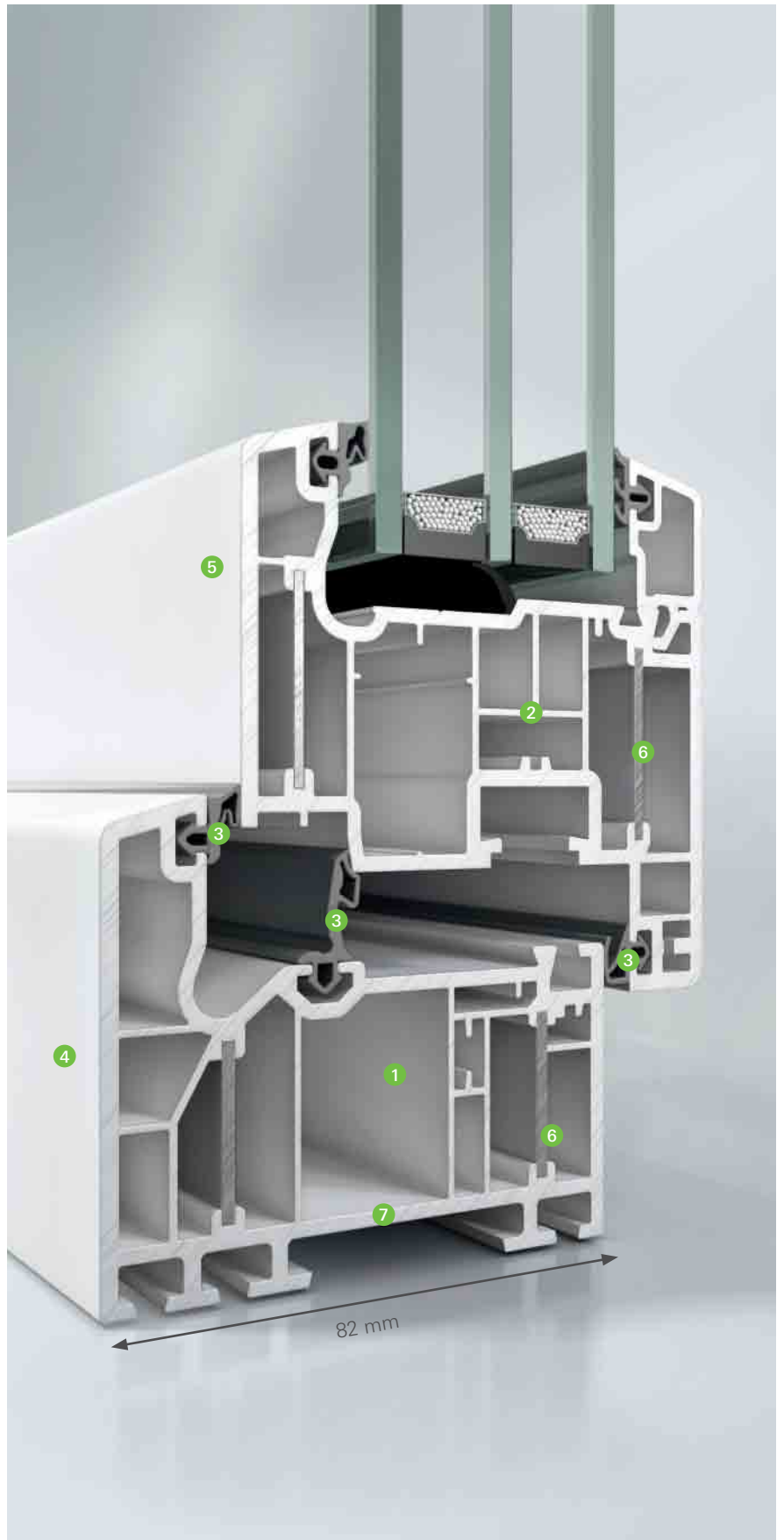
Alu Inside-Fensterprofilsystem
